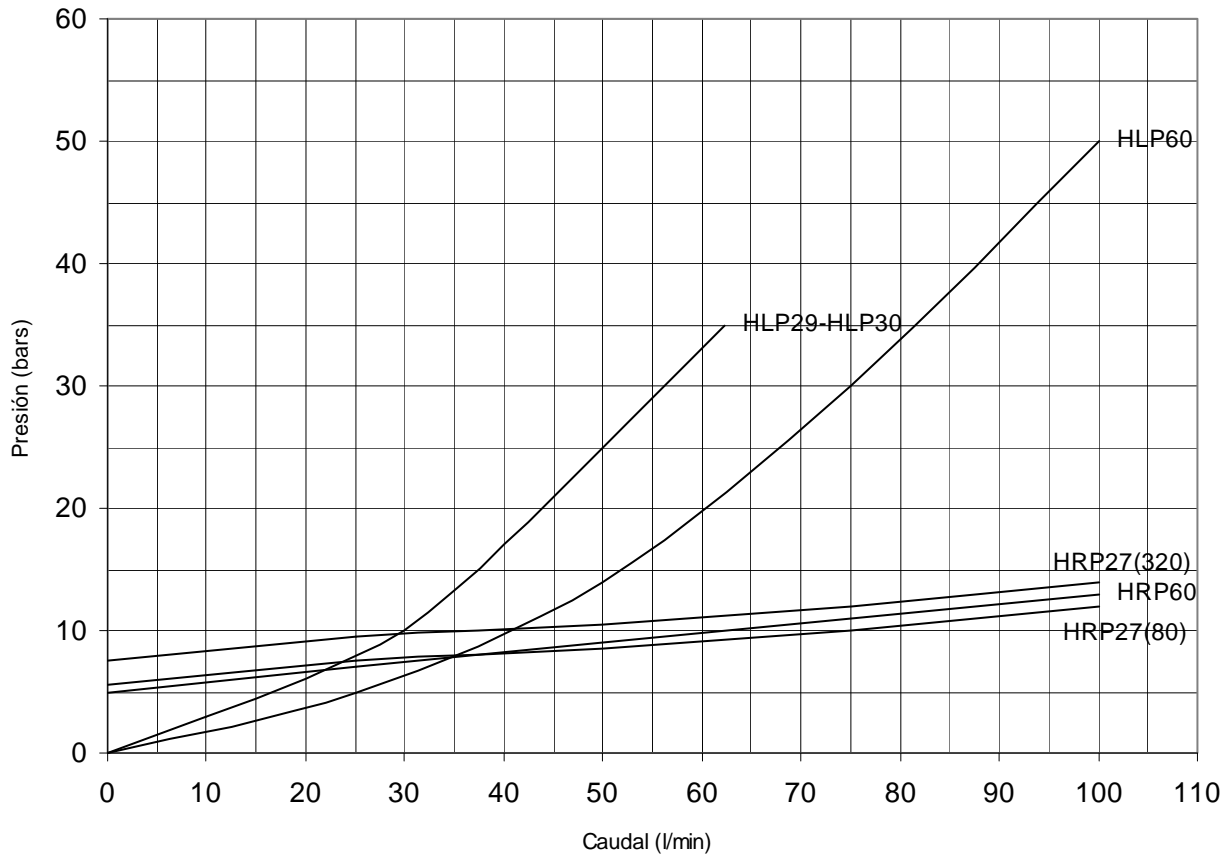
GRAFICO DE PRESIÓN MÍNIMA REGULABLE EN FUNCION DEL CAUDAL PARA CARTUCHOS LIMITADORES
