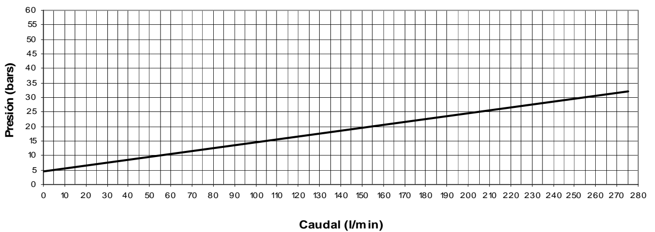
GRÁFICO DE PRESIÓN MÍNIMA REGULABLE EN FUNCION DEL CAUDAL PARA CARTUCHO LIMITADOR HRP80
